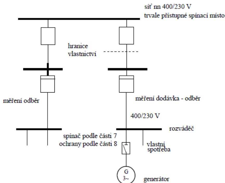
Příklad 1b Paralelně provozovaná výrobní v síti nn bez možnosti ostrovního provozu Celá výroba bez vlastní spotřeby dodaná do DS Rozšíření stávajícího odběru o výrobu
