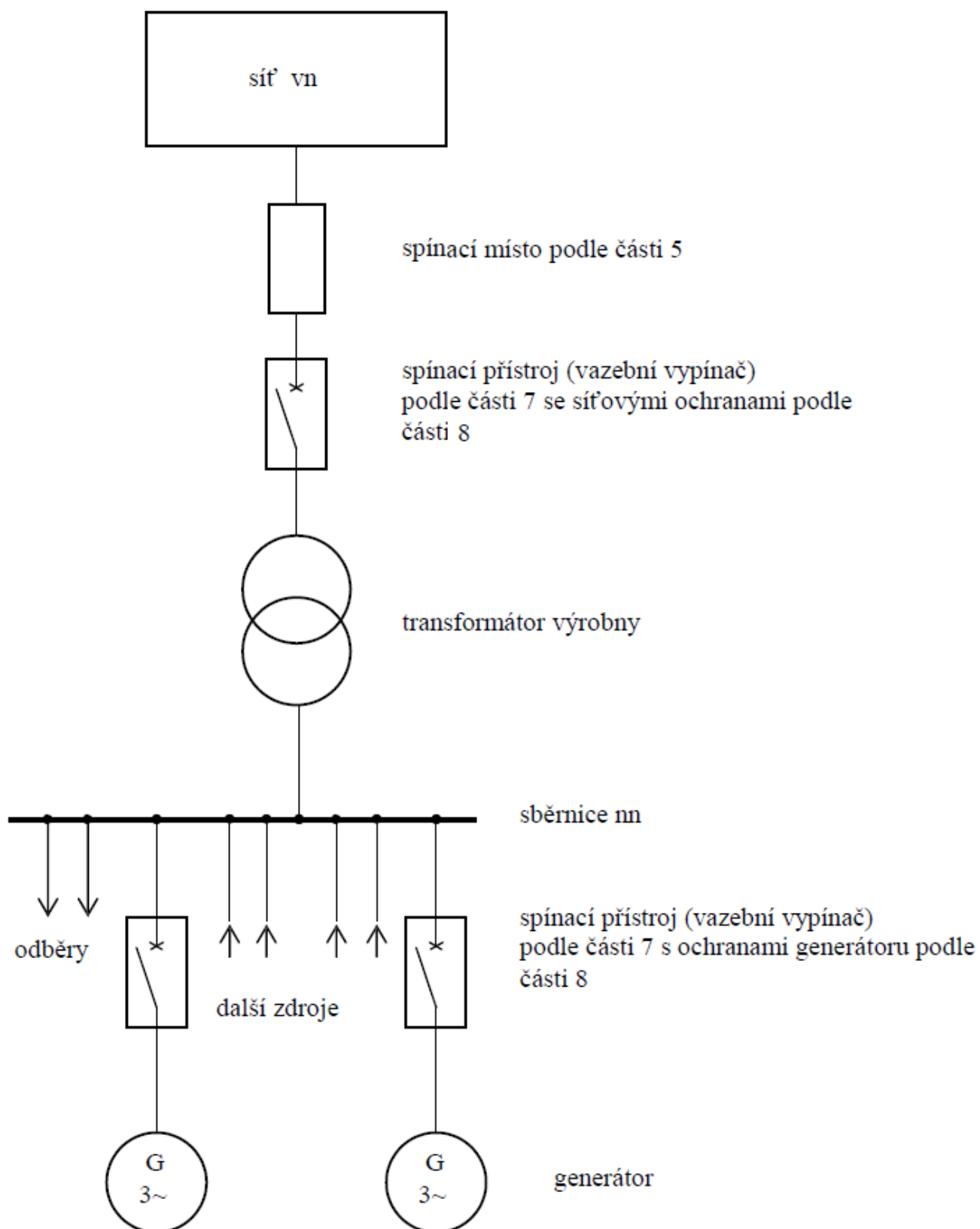
Příklad 6 Výrobna s více generátory v paralelním provozu se sítí s možností ostrovního
